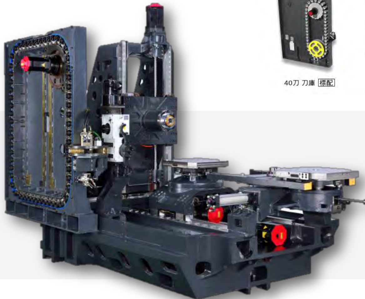
60刀 刀庫 選配
