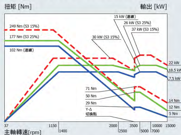
■BBT 40 / 15,000 rpm 直結驅動主軸 標配
