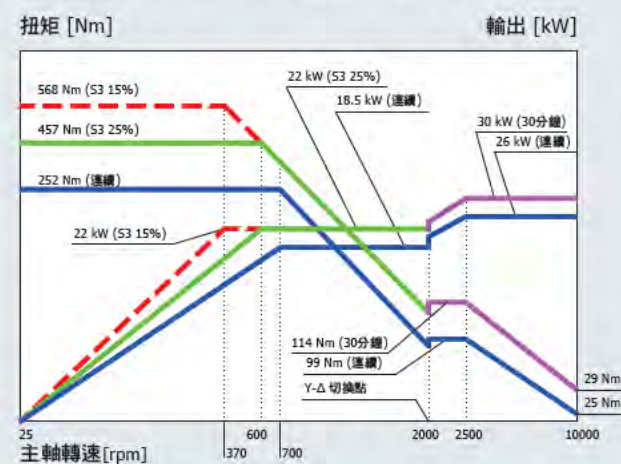
■BBT 50 / 10,000 rpm 直結驅動主軸 標配
